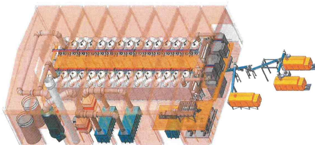
Abbildung 7: Planungsstand der Klärschlamm-Trocknungsanlage
